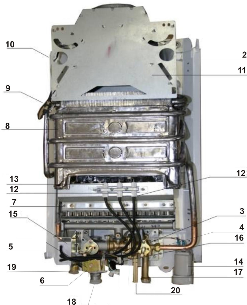
Рис. 1.1 Водонагреватель проточный газовый бытовой
